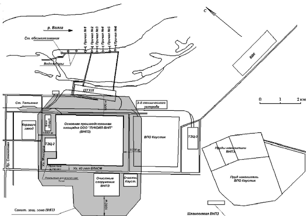
Рис. 1. Расположение производств на промышленной площадке ООО «ЛУКОЙЛ-Волгограднефтепереработка»
