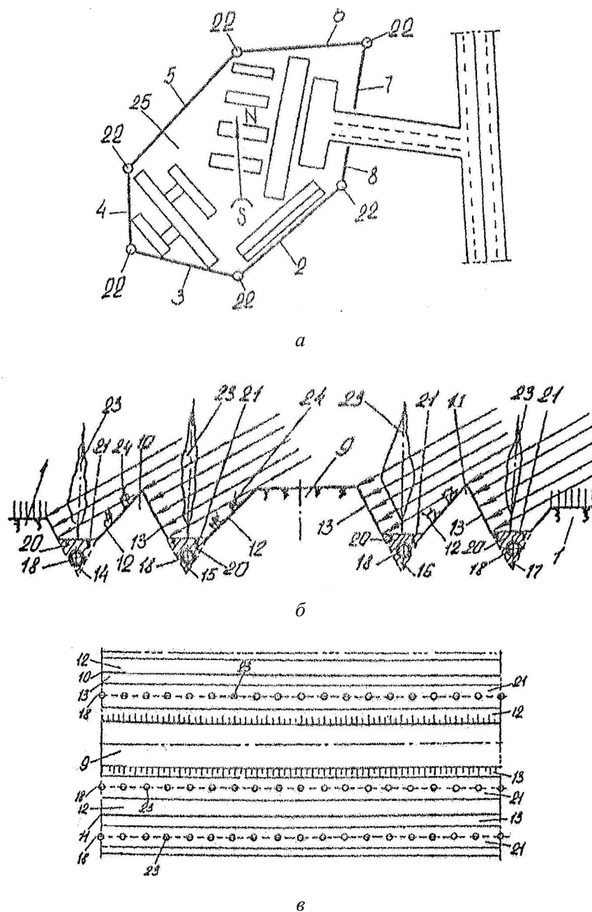
Рис. 3. Проект ограждения промышленного предприятия защитным насаждением: а – ограждение предприятия по периметру защитным насаждением, вид в плане (2–8 – участки трассы; 22 – дренажные колодцы; 25 – территория предприятия); б – поперечное вертикальное сечение предлагаемой трассы с защитными насаждениями в межгребневых впадинах (1 – верхний плодородный слой почвы; 9 – насыпное волокно технологической дороги; 10, 11 – насыпные гребни; 12, 13 – склоны гребней; 14–17 – дно канав; 18 – пластмассовые оросительные трубы; 20 – плодородный слой почвы; 21 – выровненный рельеф; 23 – саженцы деревьев; 24 – саженцы кустарников); в – то же, что б, вид в плане
